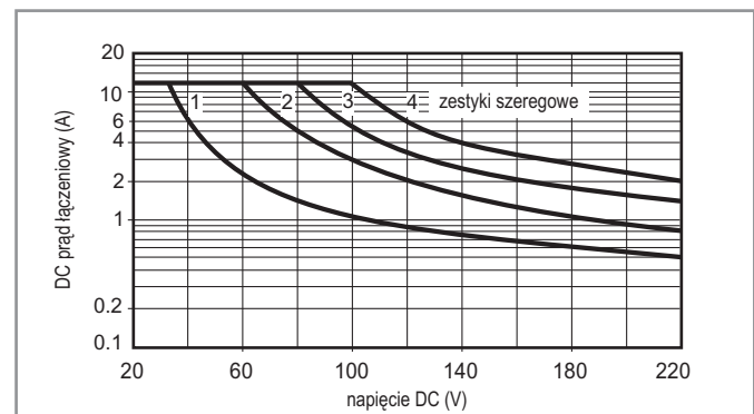
H 56 - Obciążenie graniczne dla prądu stałego (dla DC1) przy obciążeniu rezystancyjnym dla zestyków zwrotnych, przerwa zestykowa > 1,5mm
