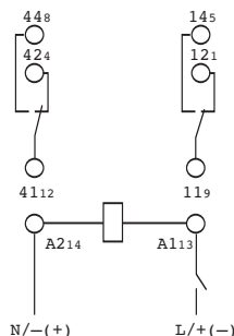
schemat połączeń
