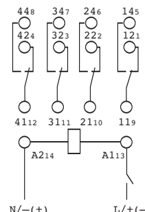
schemat połączeń
