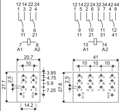
56.42 rys. otworów montażowych 56.44 rys. otworów montażowych
