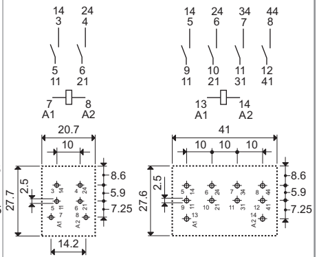
56.42-0300 rys. otworów montażowych 56.44-0300 rys. otworów montażowych
