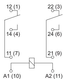
2P - przełączne
