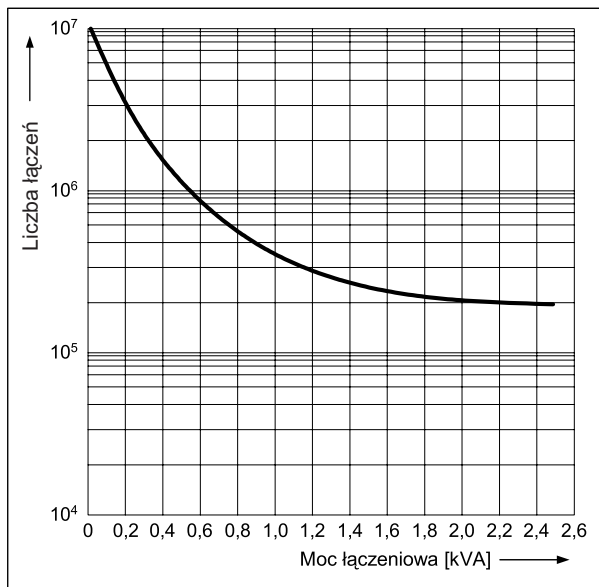
Trwałość łączeniowa w funkcji mocy obciążenia. Obwód bezindukcyjny. Maksymalna Wykres 1 częstotliwość łączeń przy obciążeniu znamionowym
