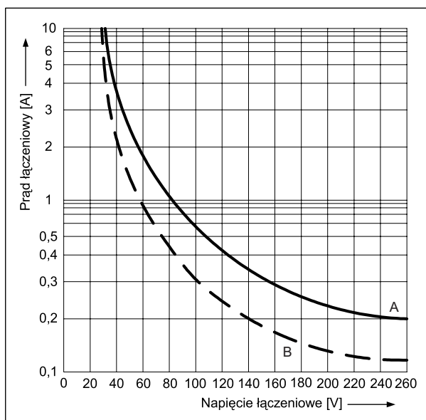
Maksymalna zdolność łączeniowa dla prądu stałego A - obciążenie rezystancyjne T = 0 ms Wykres 3 B - obciążenie indukcyjne L/R = 40 ms
