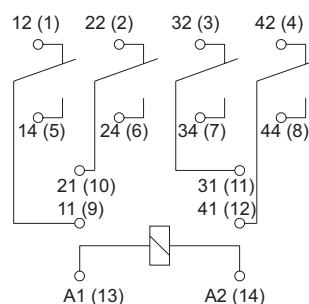
4P - przełączne
