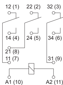
3P - przełączne
