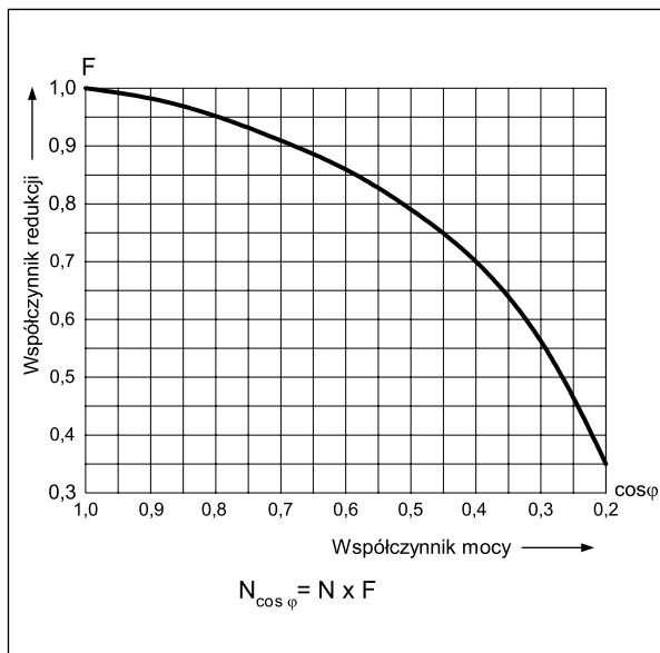
Współczynnik redukcji trwałości łączeniowej dla indukcyjnych obciążeń Wykres 2 prądu przemiennego
