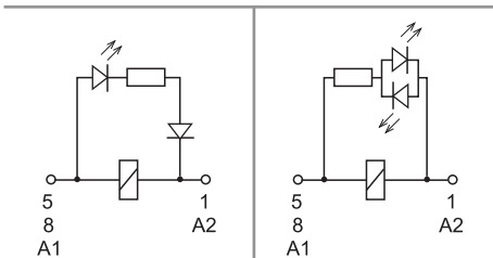
C: Opcja 54 LED (AC) C: Opcja 74 LED (DC - neutralna biegunowość)
