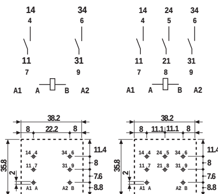
62.22 - 0300 rys. otworów montażowych 62.23 - 0300 rys. otworów montażowych
