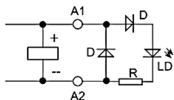
Zielony wyświetlacz LED + dioda gaszeniowa (standardowa biegunowość)
