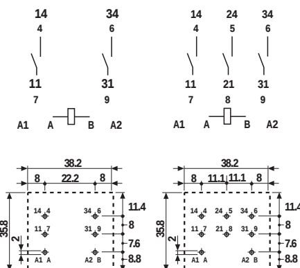
62.22 - 0300 rys. otworów montażowych
