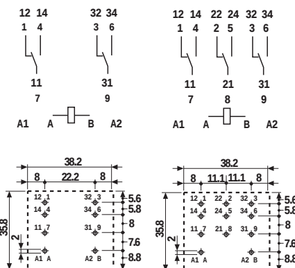
62.22 rys. otworów montażowych
