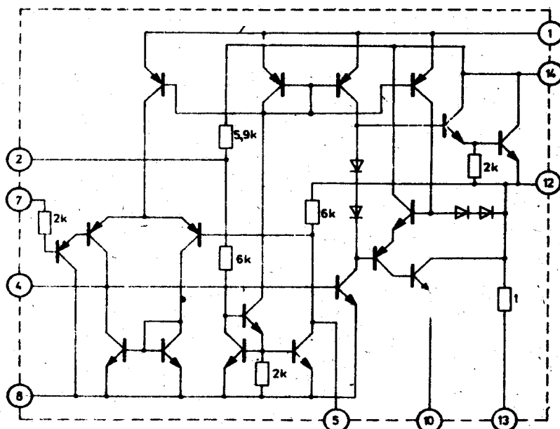
Schemał wewnętrzny
