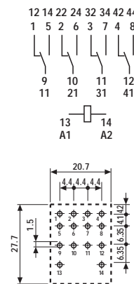
rys. otworów montażowych
