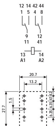
rys. otworów montażowych
