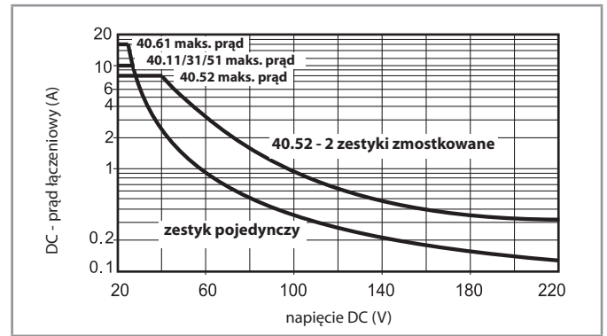
H 40 - Obciążenie graniczne dla prądu stałego (dla DC1)
