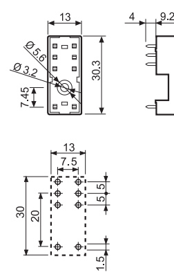
Rysunek otworów montażowych
