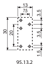
Rysunek otworów montażowych
