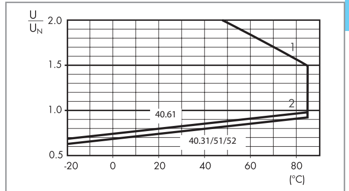
R 40 - DC Dopuszczalny zakres napięcia pracy cewki w zależności od temperatury otoczenia - Wykonanie czułe, typy 40.31/51/52/61
