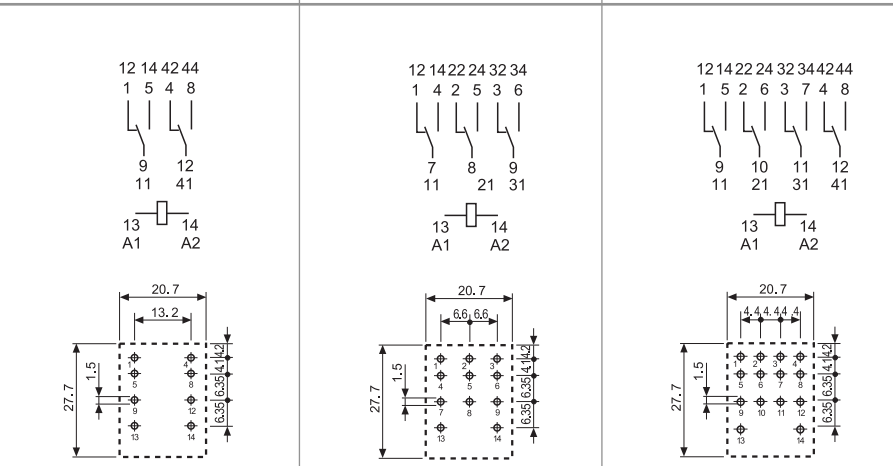
rysunek otworów montażowych
