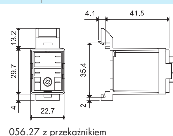
Adapter górny do montażu na szynie DIN (EN 60715) do typów 55.32, 55.33, 55.34 056.27
