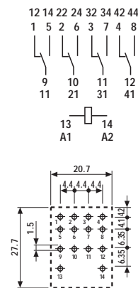
rys. otworów montażowych
