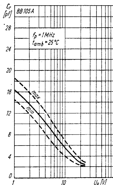
Pojemność diody BB105A w funkcji napięcia wstecznego C_r = f(U_R)
