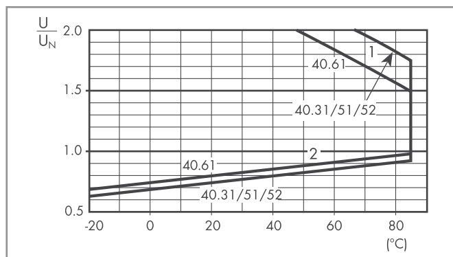
R 40 - DC - Dopuszczalny zakres napięcia pracy cewki w zależności od temperatury otoczenia Wykonanie DC czułe 500 mW (Typy 40.31/51/52/61)
